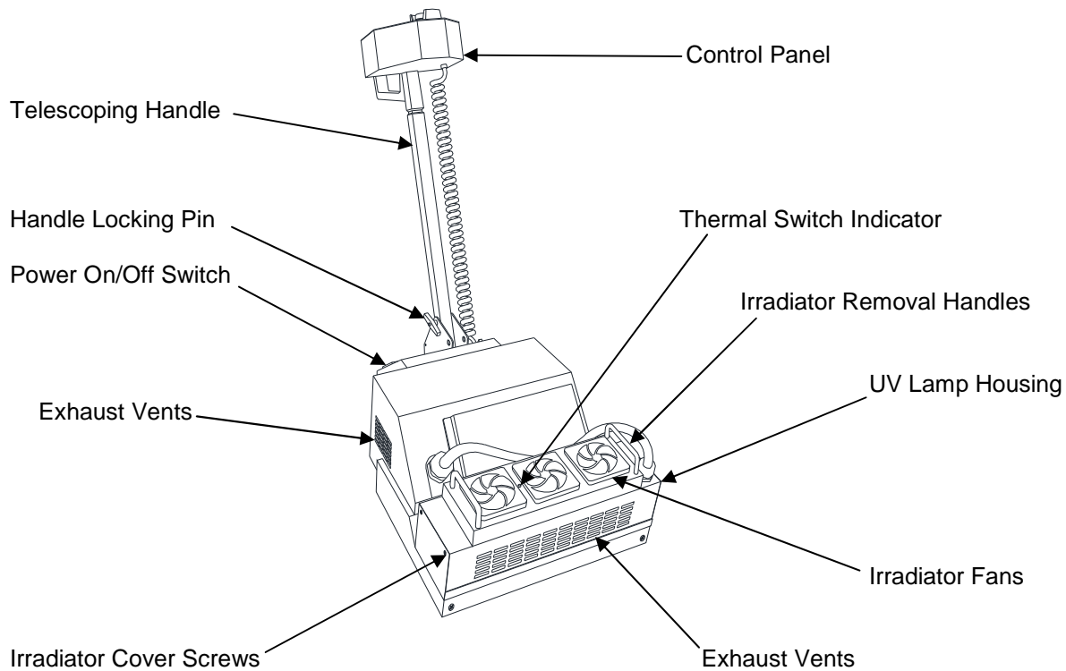
Fig. 9 Irradiator Module
